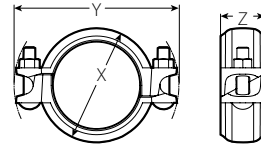
Csőkötés összeszerelve
