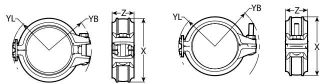
Model 109 Gemonteerde Koppeling
