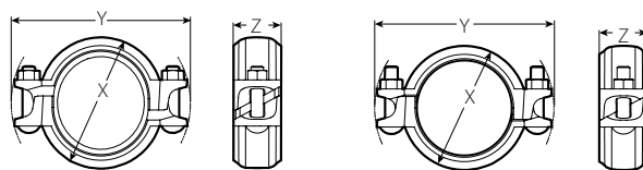
Model 009N asamblat pentru îmbinare
