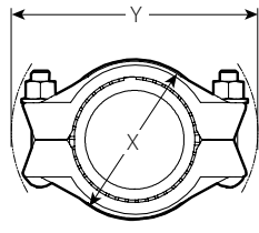
Zmontowany łącznik typu 905
