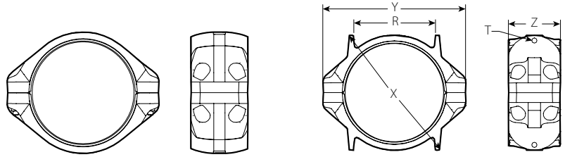
Diamètres nominaux IPS de 8 à 18 po et ISO de 250 à 450mm
