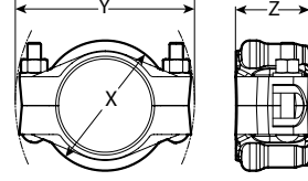
Stil 907 Hazır Monte Bağlantı
