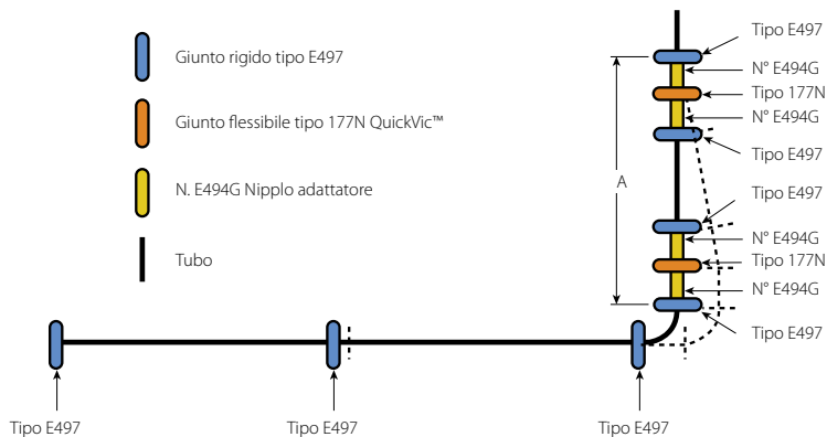
Esempio di giunto flessibile di tipo 177N QuickVic™ con capacità di deflessione
