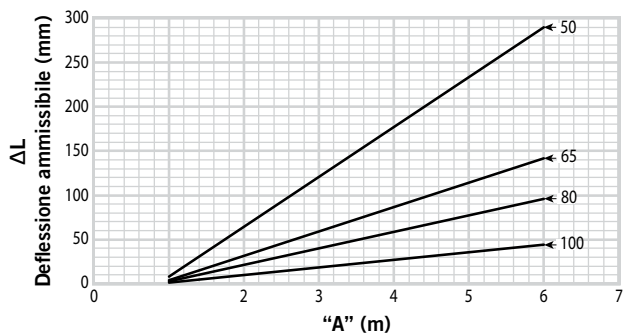
Movimento di StrenghThin™ 100 – "sottile" 2 – 6"/DN50 – DN150: Spessore della parete ≤ 2,3 mm
