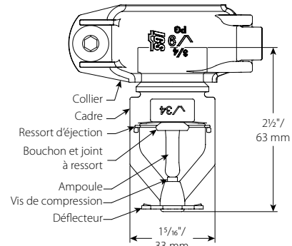
Rainuré V3407
