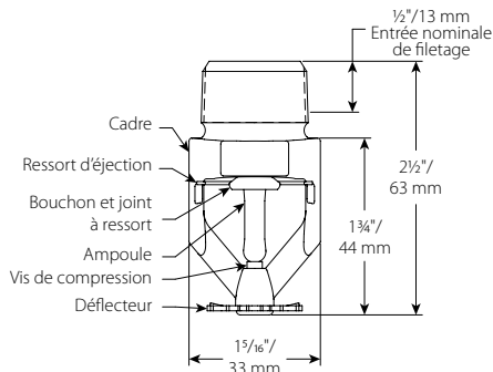
Fileté V3407
