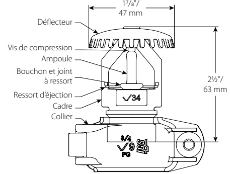
Rainuré V3403
