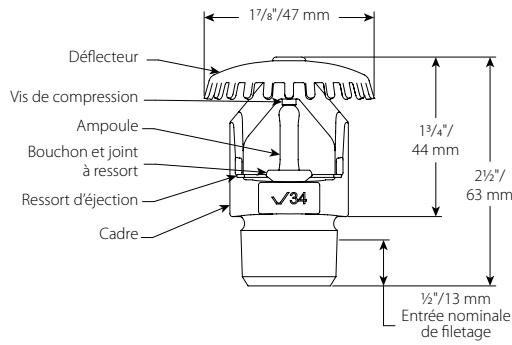
Fileté V3403
