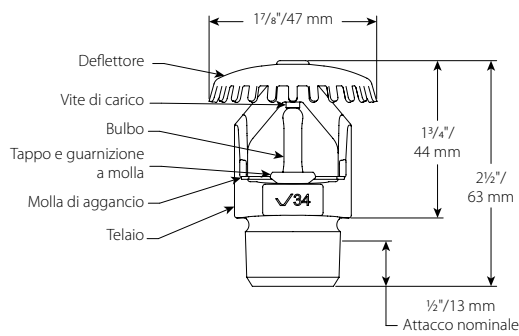
Filettato V3403
