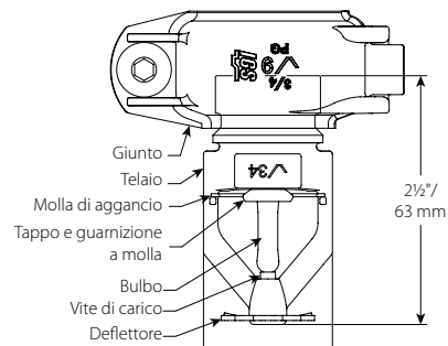
Scanalato V3407
