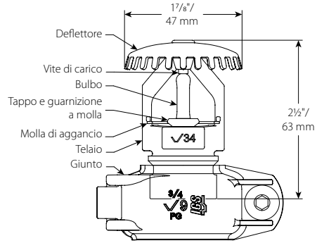
Scanalato V3403
