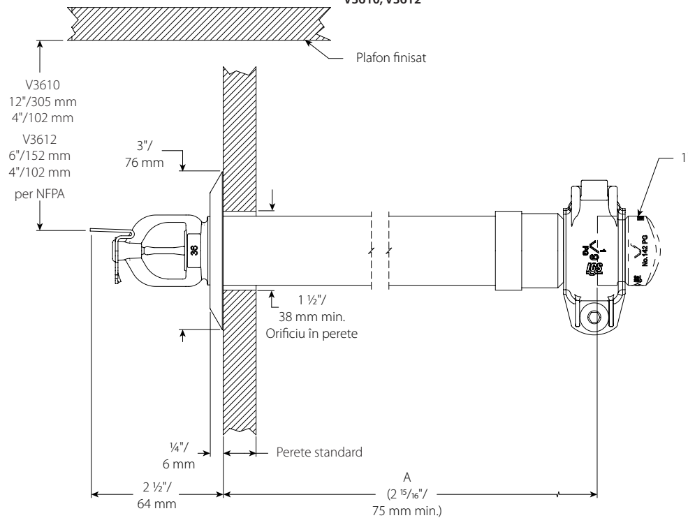
Drept, canelat V3610, V3612
