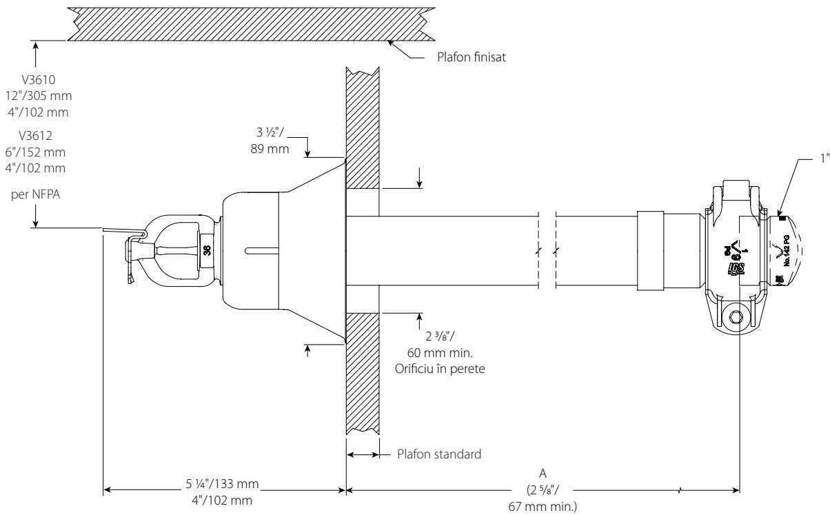
Extins, cu manșon și jupă, canelat V3610, V3612
