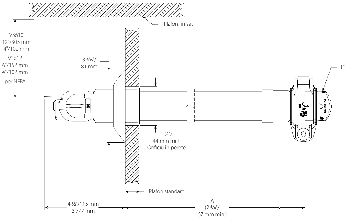
Manșon și jupă, canelat V3610, V3612
