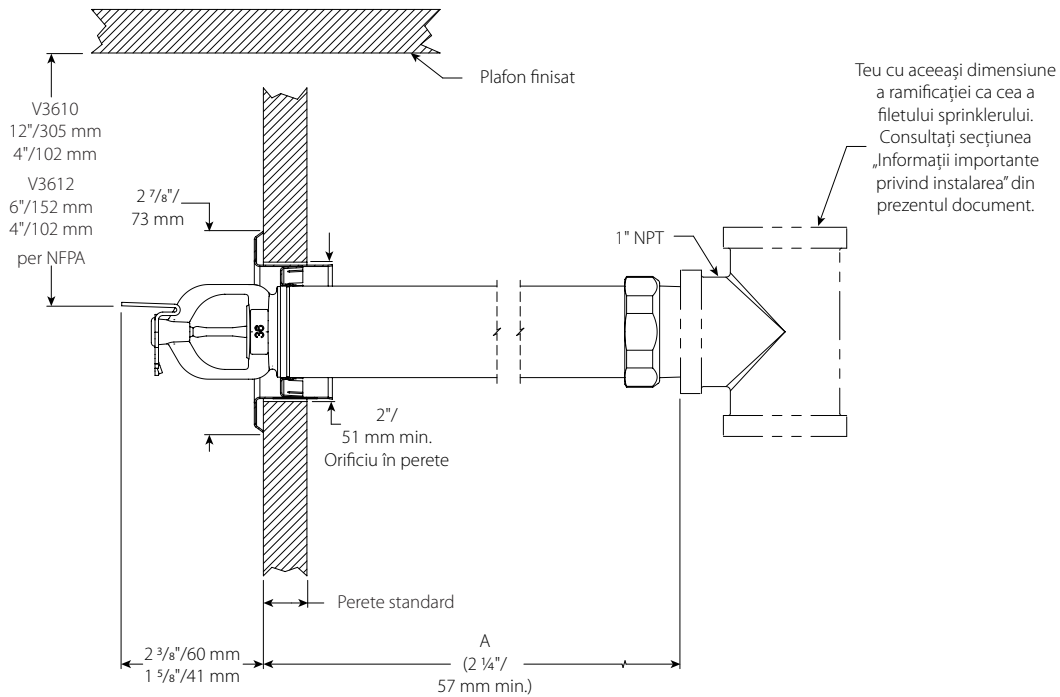
Ascuns, filetat V3610, V3612
