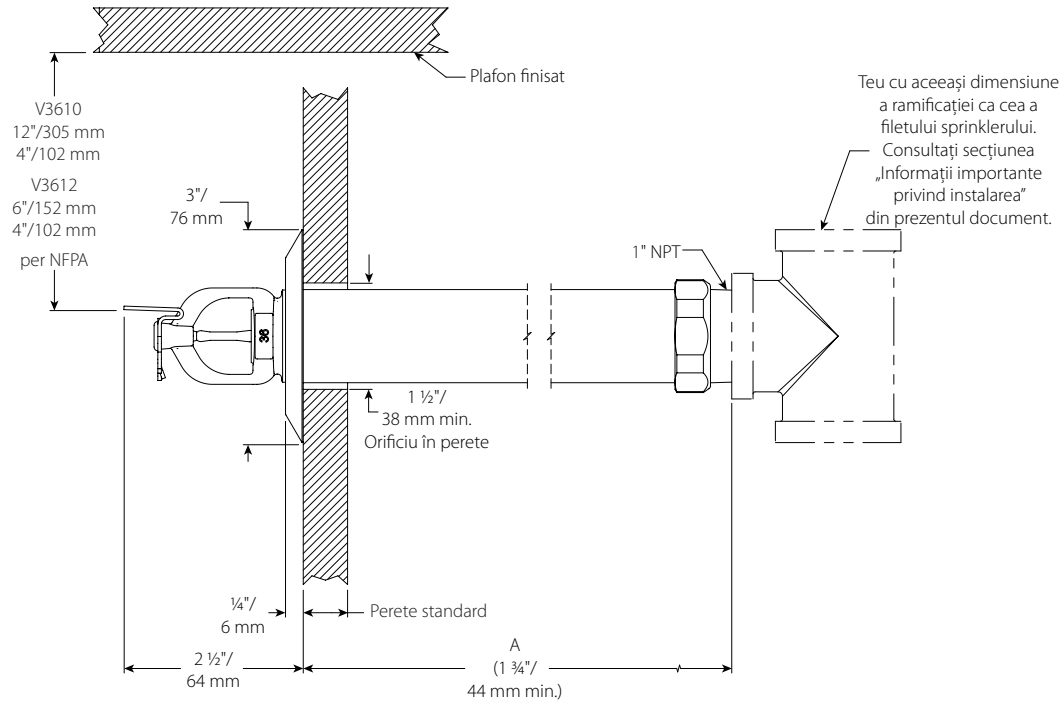
Drept, filetat V3610, V3612
