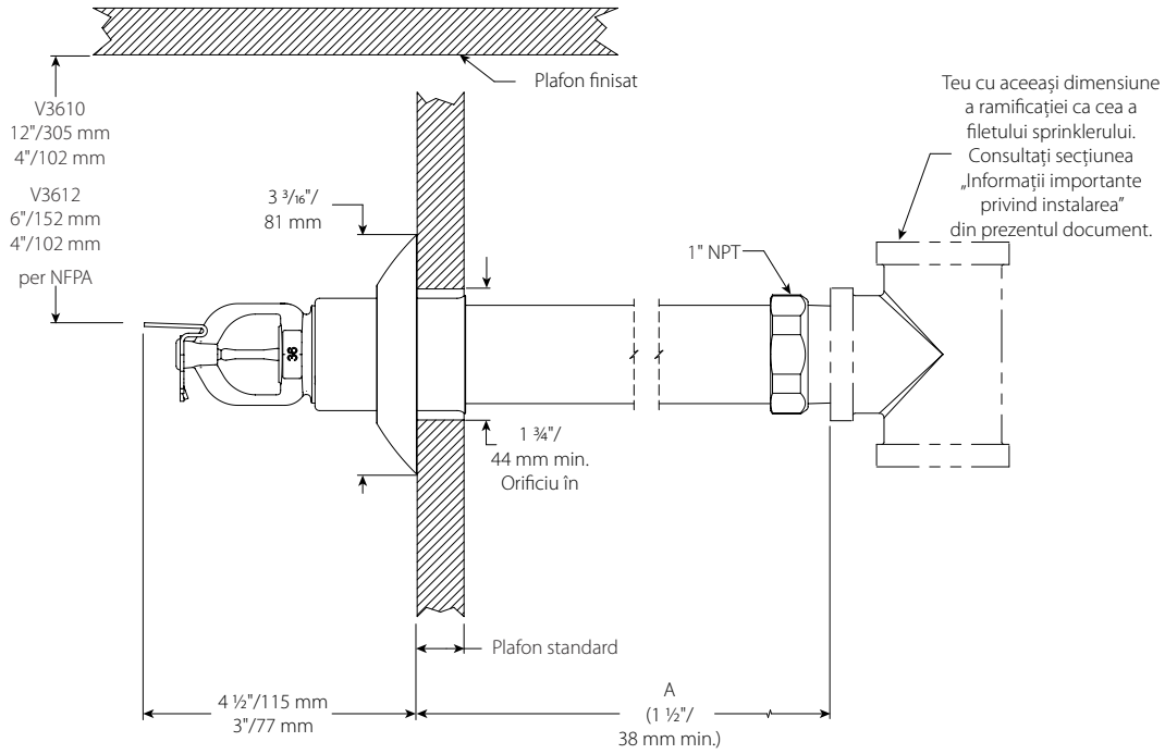
Manșon și jupă, filetat V3610, V3612
