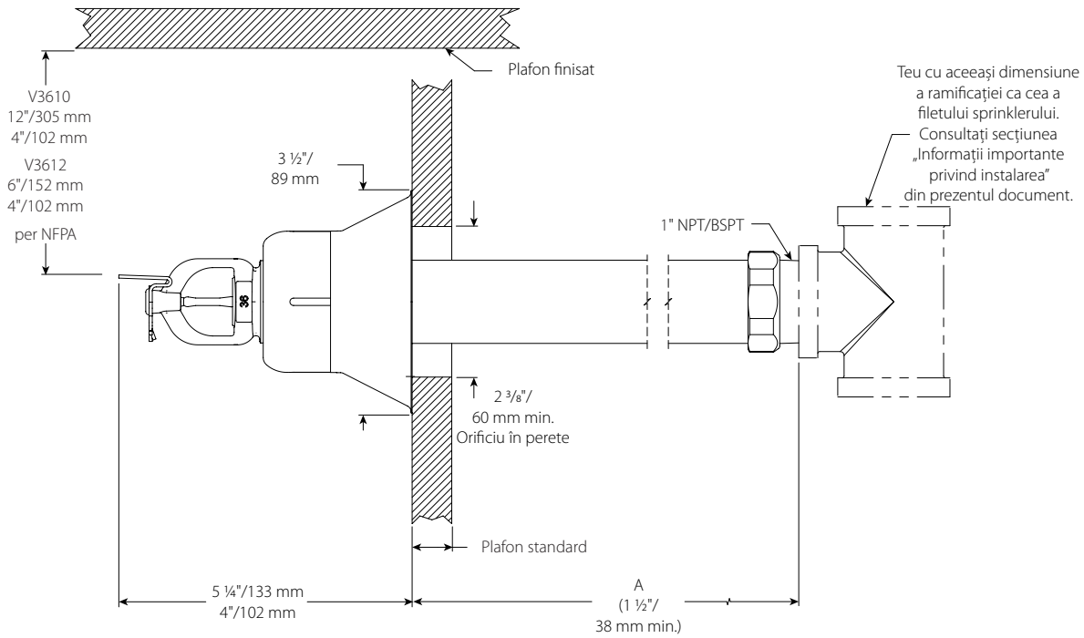
Extins, cu manșon și jupă, filetat V3610, V3612
