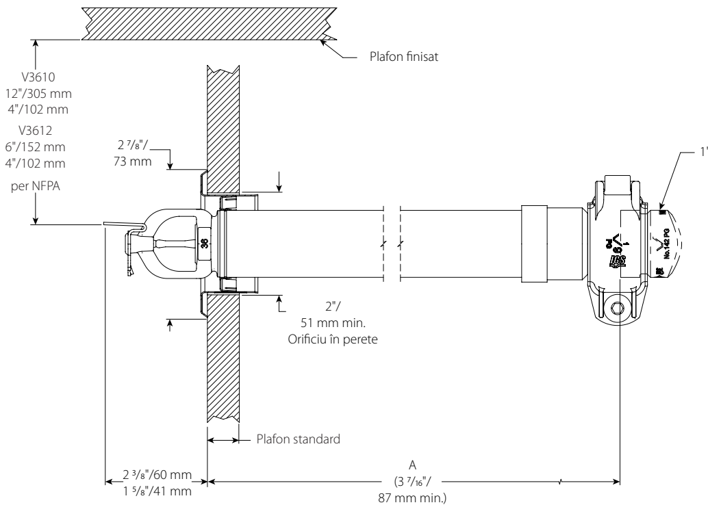
Ascuns, canelat V3610, V3612
