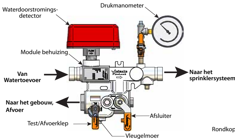
Maten 1 1/4 – 2-inch/42,4 – 60,3-mm
