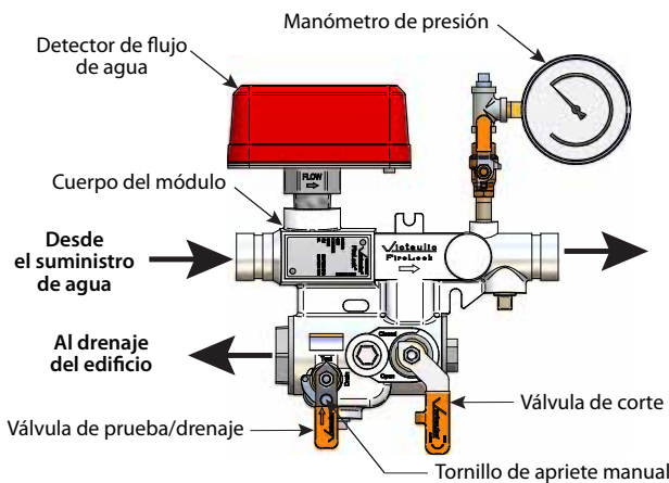
Tamaños de 1 ¼ - 2 pulg./42,4 - 60,3 mm
