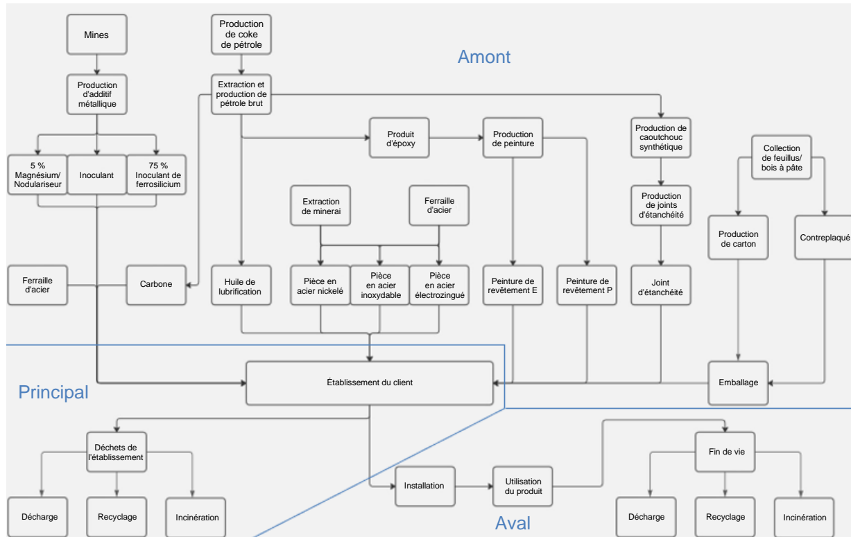
Figure 1 Diagramme des débits pour la fabrication de 1 000 kg de produit Victaulic
